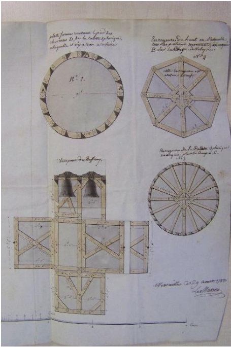
Plans de la charpente
